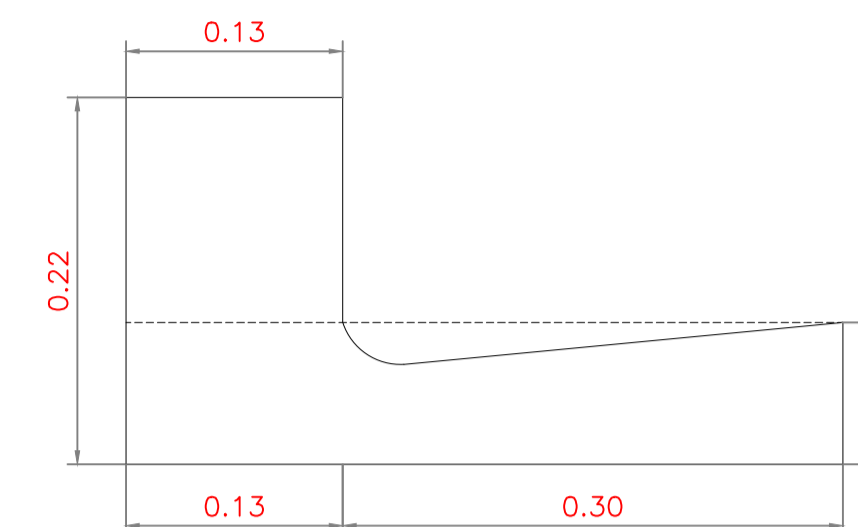
CORTE GUIAS E SARJETAS A IMPLANTAR S/ ESCALA
