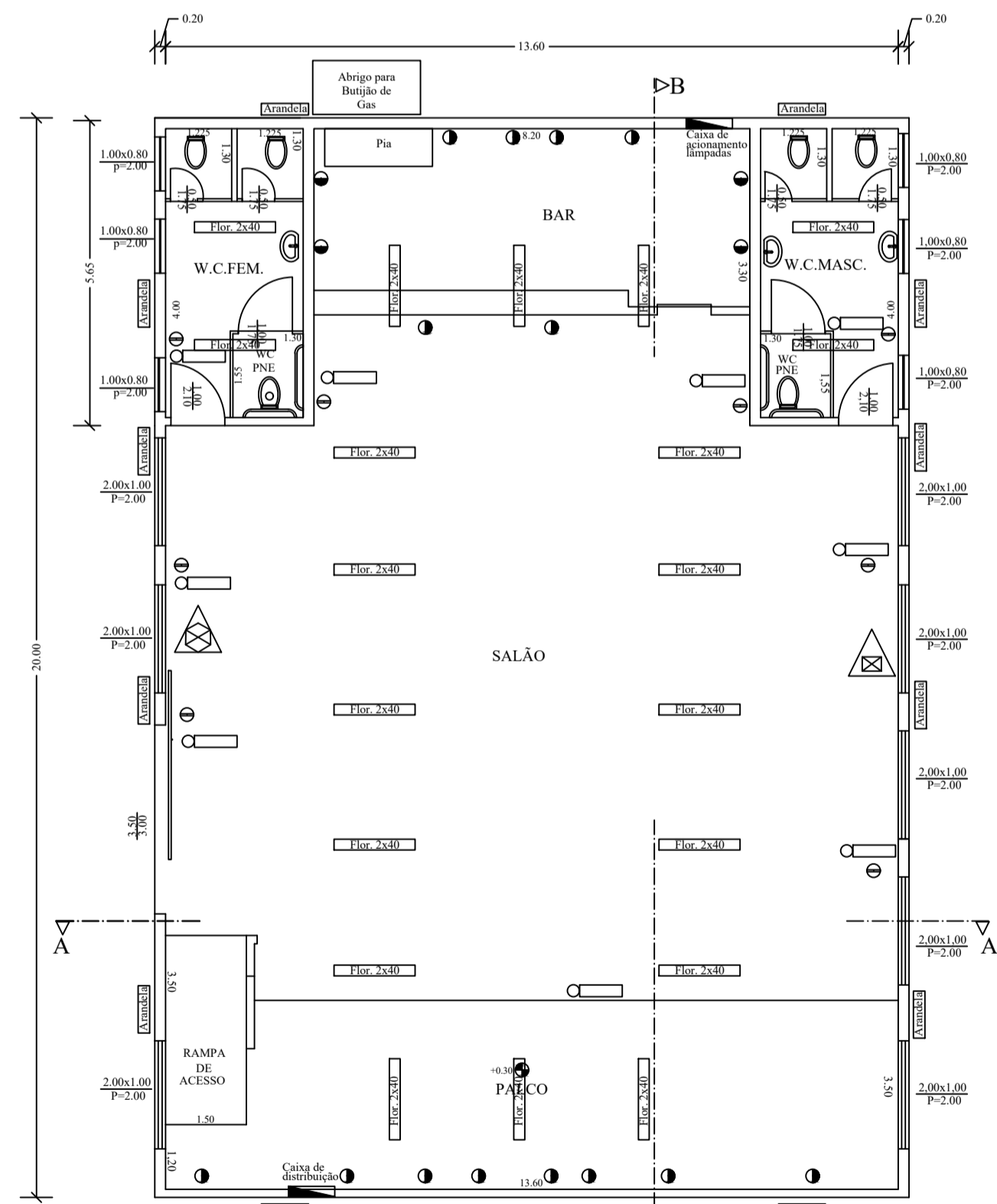
PLANTA BAIXA ESCALA--1:100 RUA DEPUTADO PLÍNIO SALGADO
