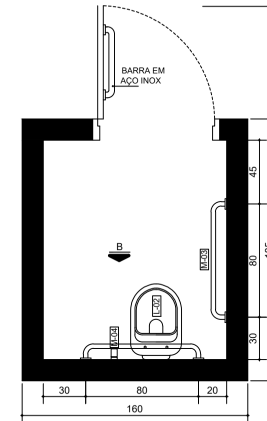
PLANTA - WC ADAPTADO P/ PORTADORES DE NECESSIDADES ESPECIAIS SEGUNDO NBR 9050/2004 ESC. 1:25
