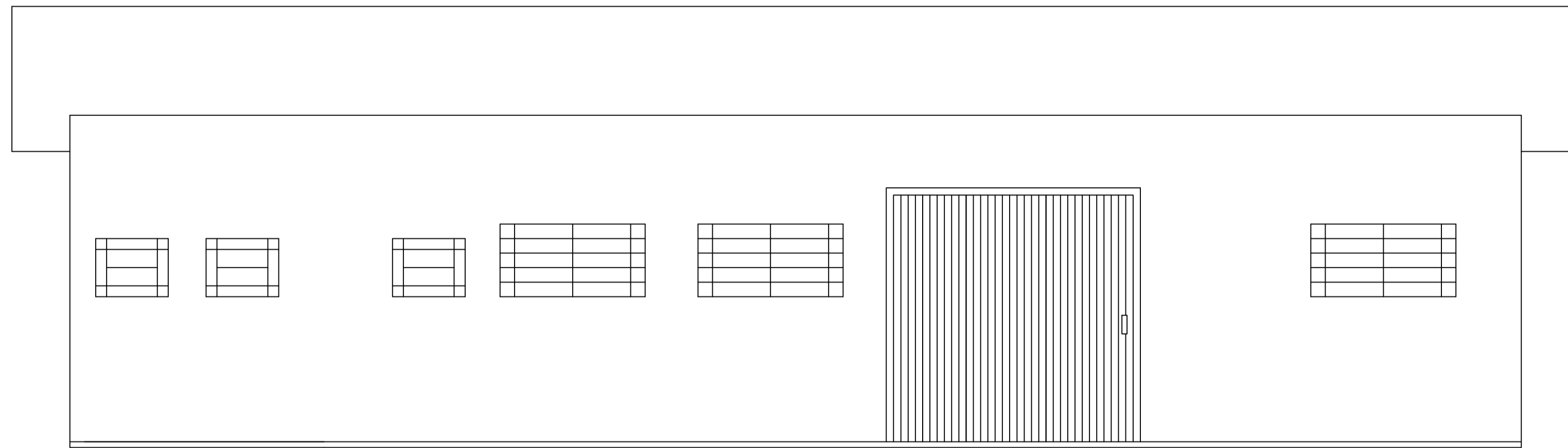
FACHADA (AVENIDA CLODOMIRO NEGRINI) ESCALA--1:50
