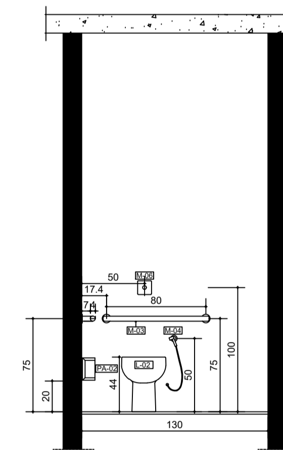
VISTA B - LAVABO MASCULINO ESC. 1:25
